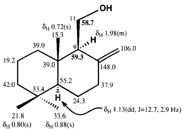
albicanol (8)
