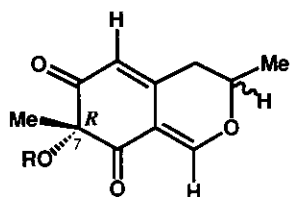
Daldinin B (82)
